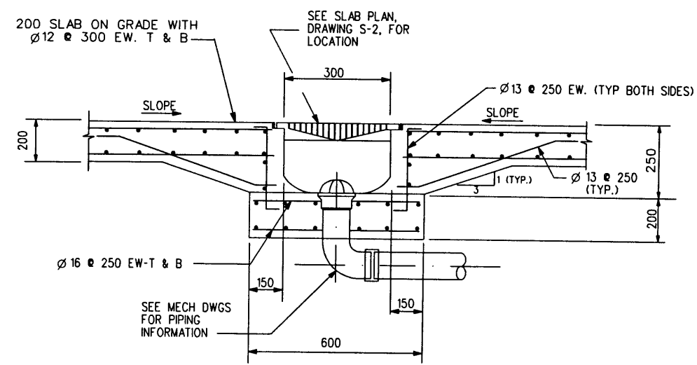
SECTION N.T.S.
