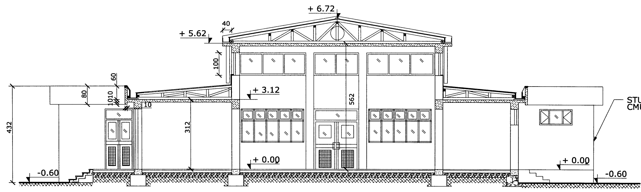
BUILDING SECTION A-A SCALE: 1:50
