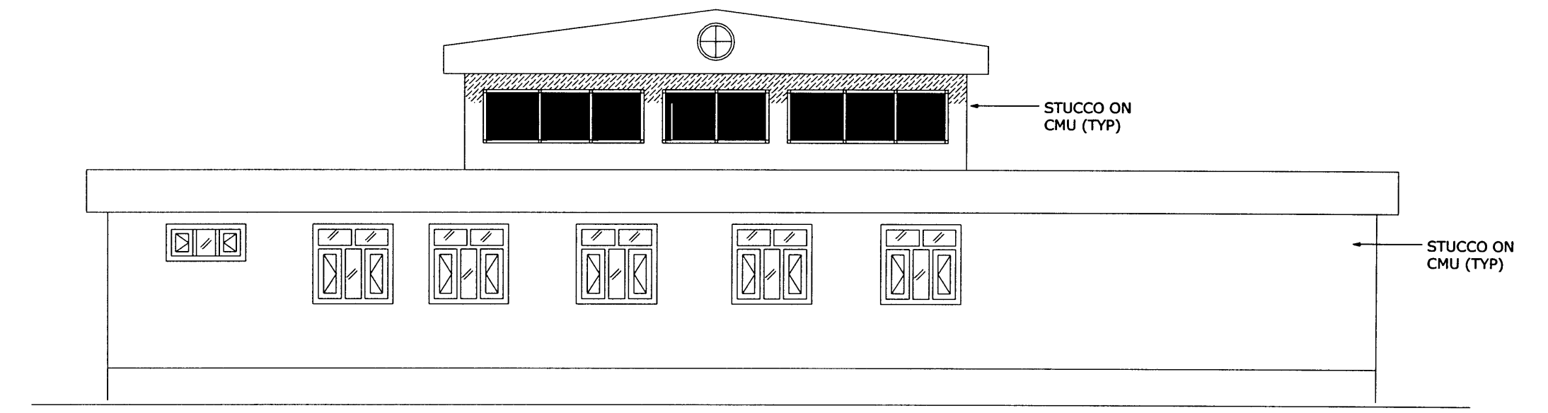
ELEVATION SCALE 1:50 B A-1A-5
