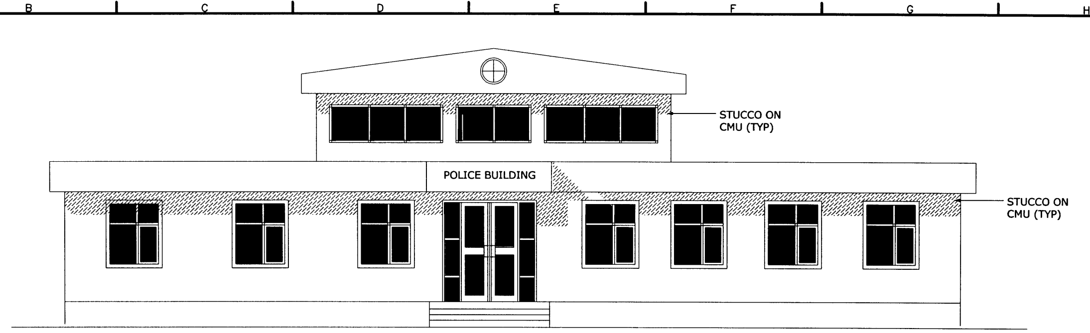
ELEVATION SCALE 1:50 A A-1A-5
