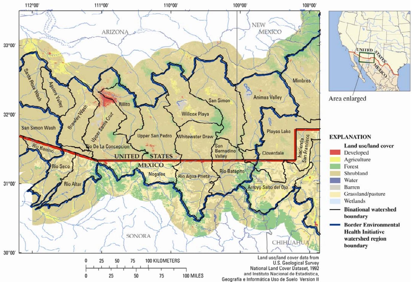
Figura 4. Área piloto para el desarrollo de cuencas hidrográficas binacionales y redes hidrográficas de la región fronteriza. El área geográfica mostrada está a lo largo de los estados fronterizos de Arizona y Sonora. Los conjuntos de datos binacionales de cobertura y uso de la tierra se usan como información de fondo.
