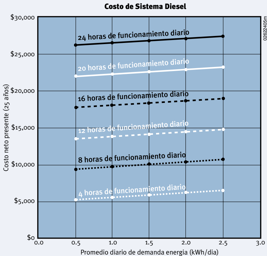
Figura 3.3. Este gráfico muestra el costo presente neto de 25 años del uso de un generador diesel. Las dos variables son el promedio diario del costo (kWh/día) y las horas de funcionamiento diario. Note que los costos solamente varían ligeramente con la carga, pero sube rápidamente con el aumento de las horas de funcionamiento.
