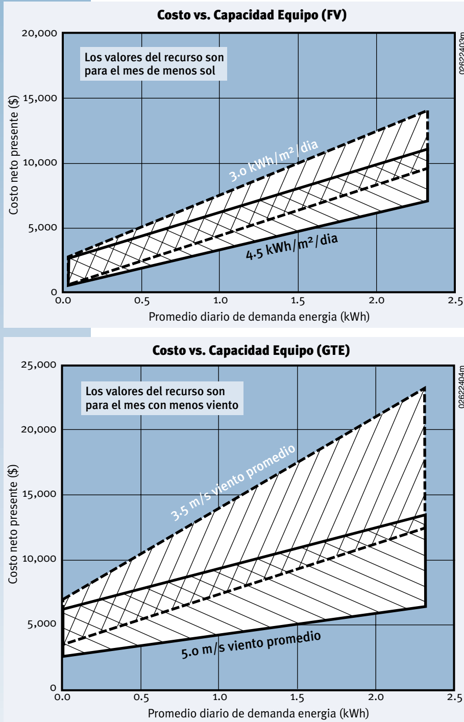
Figura 3.2. Estos gráficos muestran el rango de costo típico de la tecnología incluida (fotovoltaica o turbinas eólicas) para un sistema como una función del promedio de carga diaria. La disponibilidad de recurso incluida (para viento y para sol) es el mes con la menor disponibilidad de recurso.
