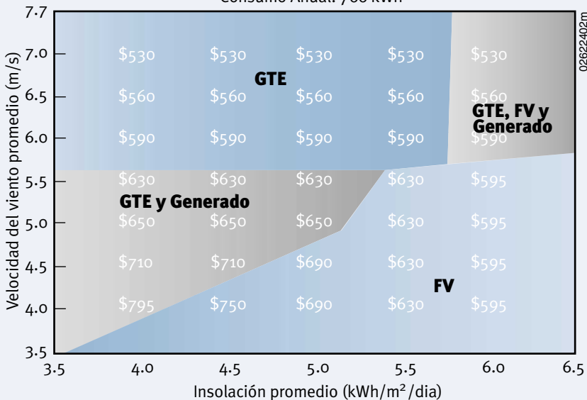
Figura 3.1. Estos gráficos muestran las configuraciones de bajo costo para dos servicios de salud de diferentes tamaños como una función del promedio de la velocidad del viento y el promedio de insolación. Los costos dados son los costos anualizados ($US/año) del sistema del menor costo con los recursos de viento y sol dados. Los resultados asumen una variación particular de supuestos económicos. Esta misma variación de información de velocidad de viento e insolación se usó para todas las opciones y escalas para obtener varios valores de promedios anuales mostrados. Los resultados intentan mostrar solamente tendencias generales. FV = fotovoltaicos, GTE = generador de turbina eólica.
