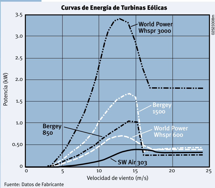
Figura 2.4. Curvas de Energía de Turbinas eólicas Selectas
