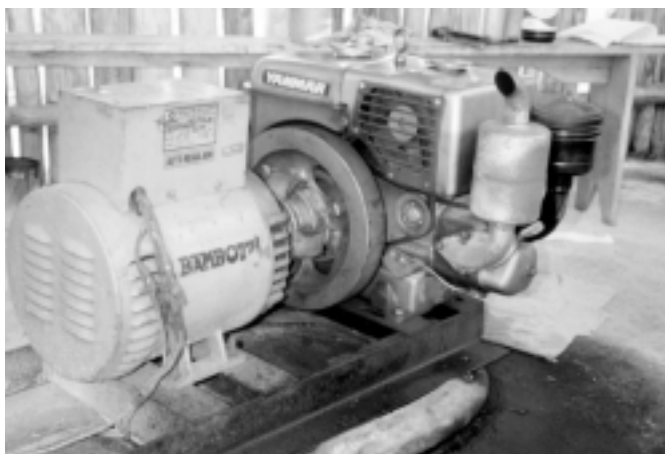
Figura 2.5. Un generador diesel es generalmente la típica fuente de energía en pequeños hospitales rurales. Las clínicas más pequeñas pueden confiar en los generadores más pequeños a gasolina solamente para usos de emergencias.
