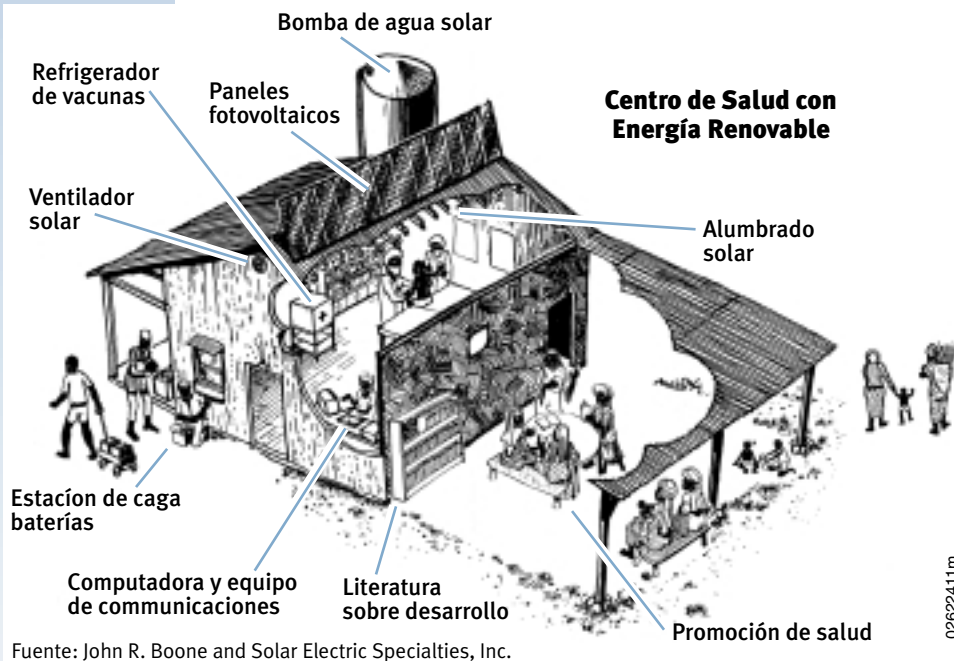
Figura 1.1. Clínica de Salud mostrando las Aplicaciones Típicas.
