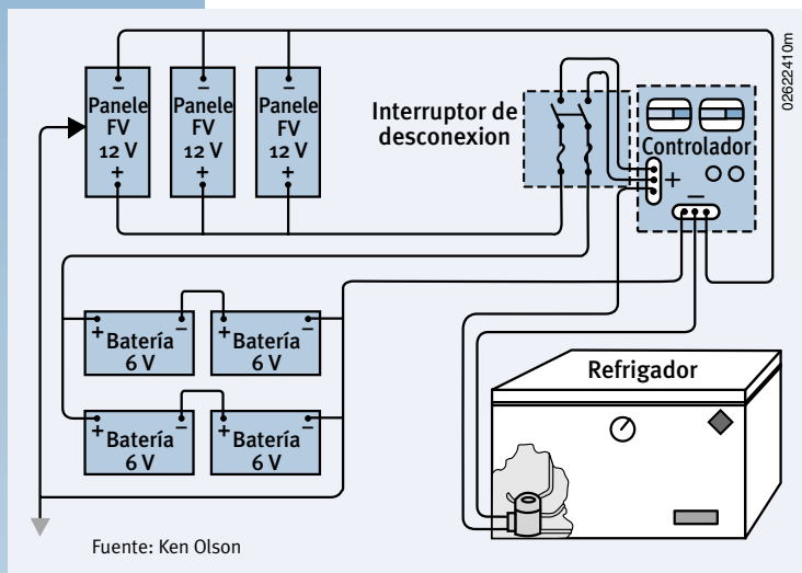
Figura 5.2. Bloque diagrama del sistema
