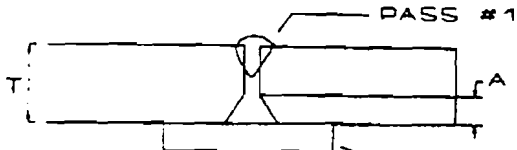
DETAIL 1A
