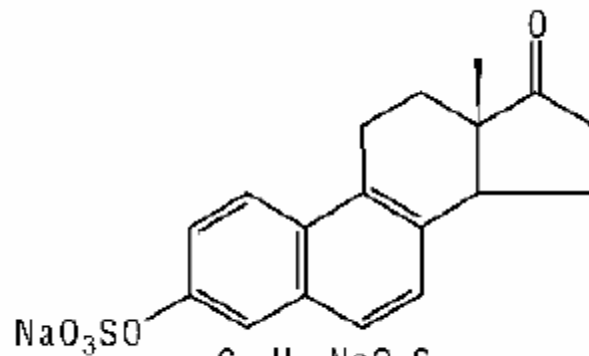
Sodium Equilenin Sulfate
