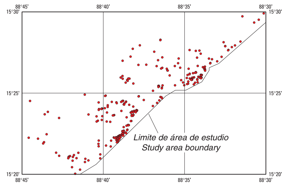
Mapa mostrando la distribución de deslizamientos de tierra en este cuadrángulo. Los puntos rojos muestran el final de la inclinación ladera arriba de cada deslizamiento de tierra. Hay 281 deslizamientos de tierra en este mapa.
