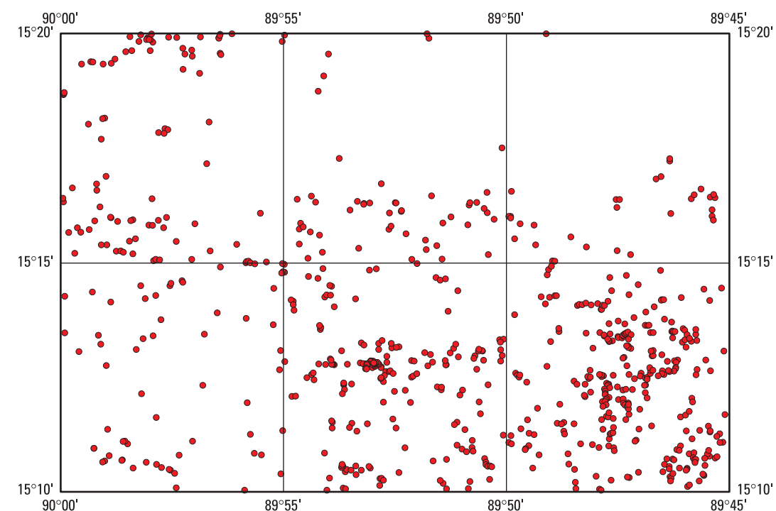
Mapa mostrando la distribución de deslizamientos de tierra en este cuadrángulo. Los puntos rojos muestran el final de la inclinación ladera arriba de cada deslizamiento de tierra. Hay 729 deslizamientos de tierra en este mapa.
