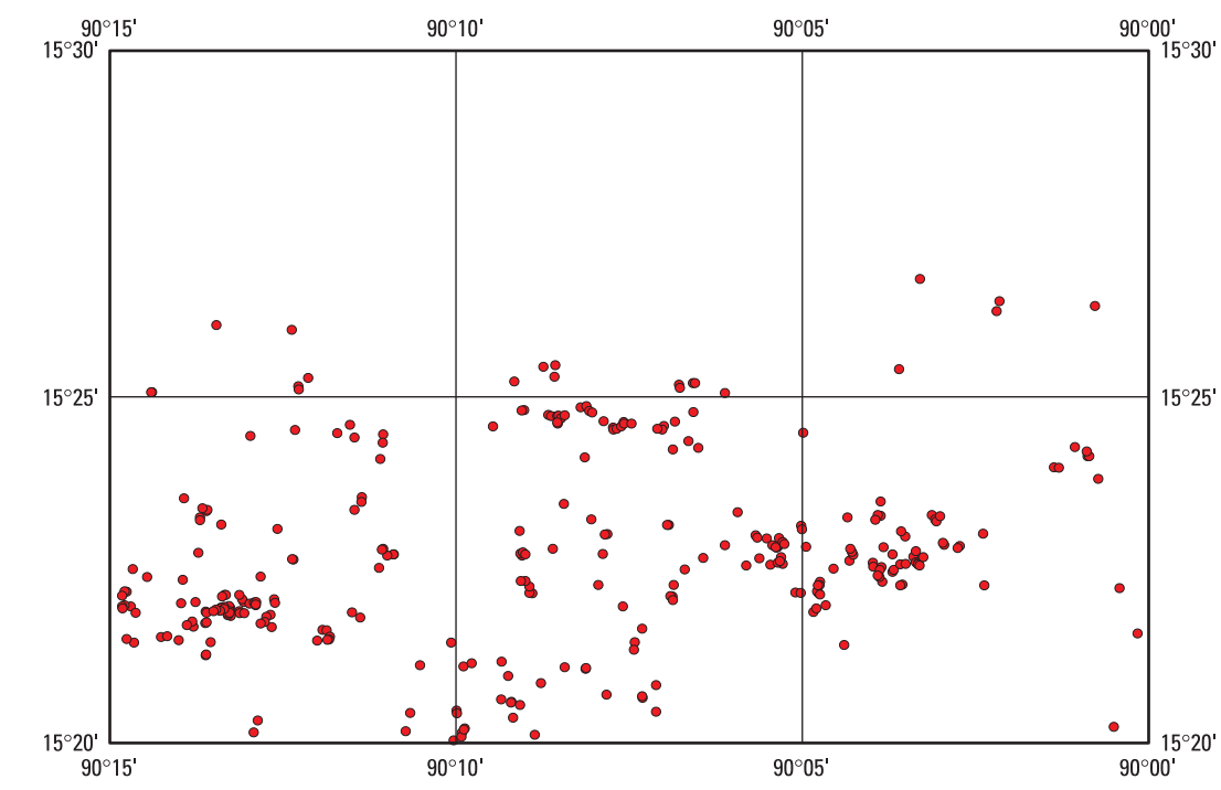
Mapa mostrando la distribución de deslizamientos de tierra en este cuadrángulo. Los puntos rojos muestran el final de la inclinación ladera arriba de cada deslizamiento de tierra. Hay 303 deslizamientos de tierra en este mapa.
