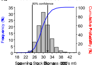
A6 Precision of 2000 SSB Estimate
