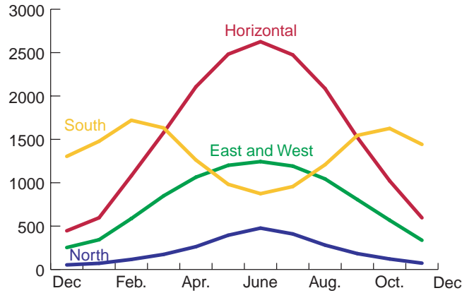
Comparison of Window Orientations — 48° Latitude
