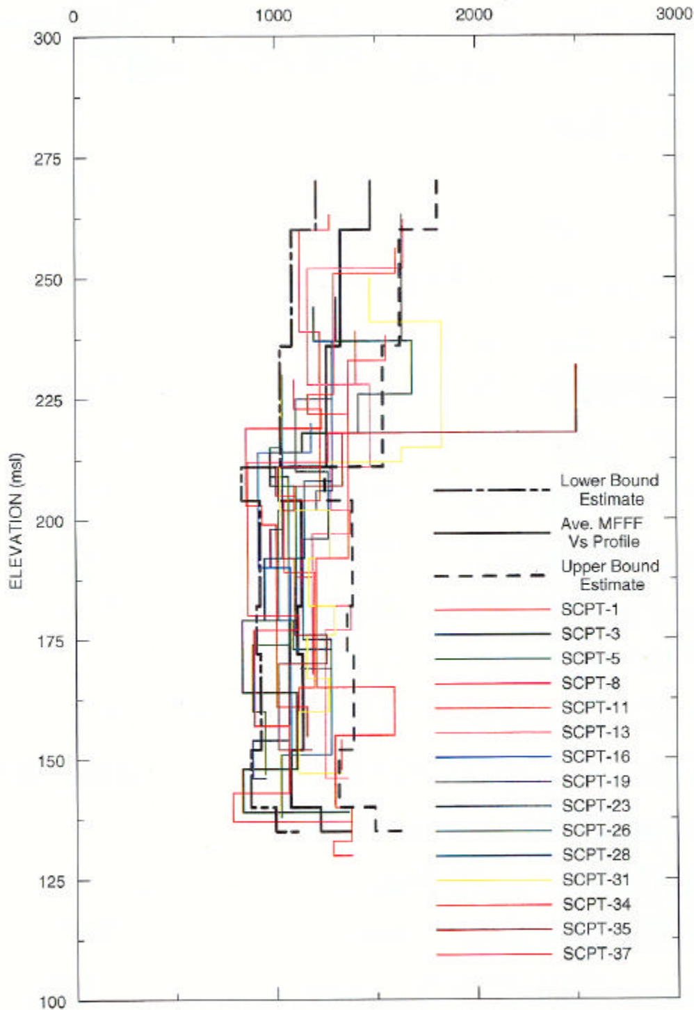
Fig 6-2-8.gr w/Shear_Wave_Values.xls 8/5/01
