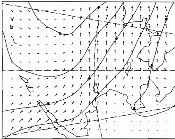
00Z 4 MAR 1981
