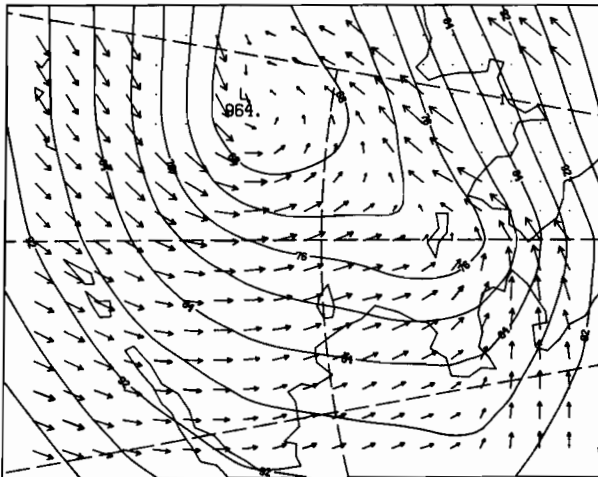
00Z 2 MAR 1981
