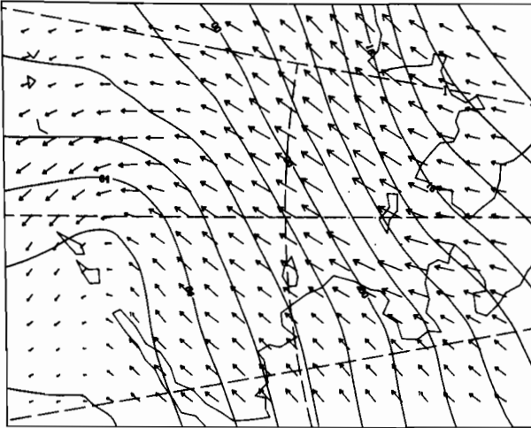
00Z 9 MAR 1981
