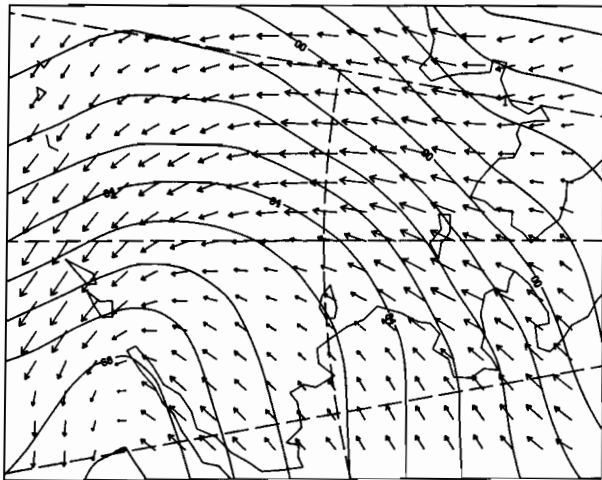
00Z 14 MAR 1981
