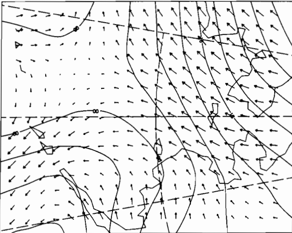
00Z 11 MAR 1981
