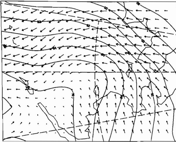
00Z 15 MAR 1981
