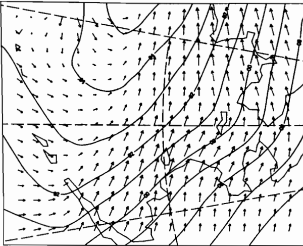
00Z 18 MAR 1981
