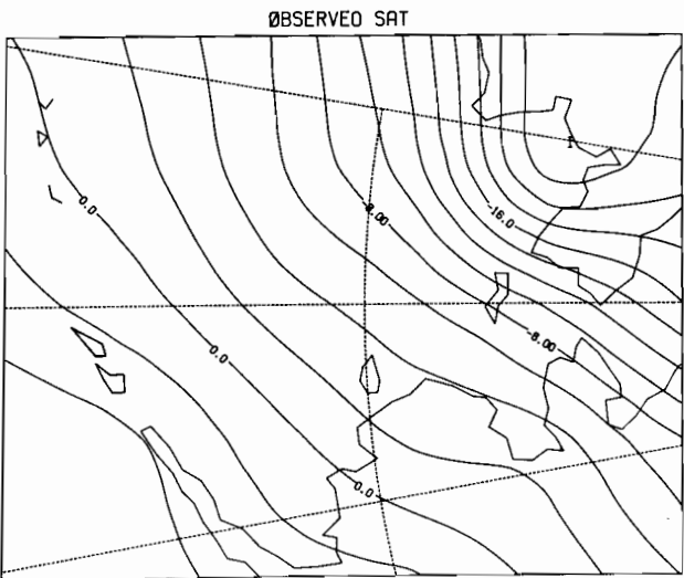
00Z 8 MAR 1981
