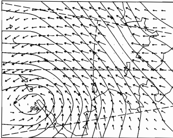
00Z 13 MAR 1981
