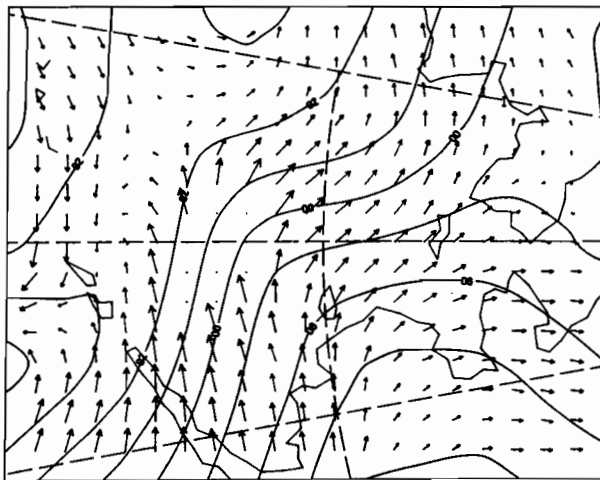
00Z 20 MAR 1981
