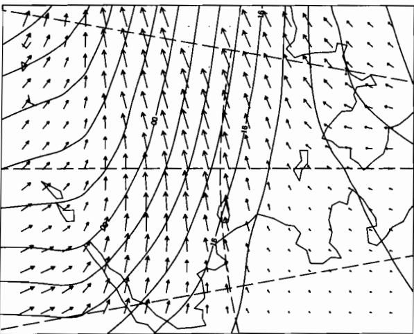
00Z 24 FEB 1981
