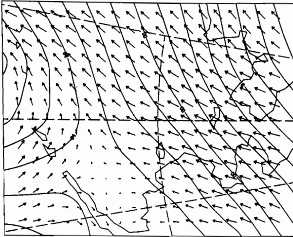
00Z 12 MAR 1981
