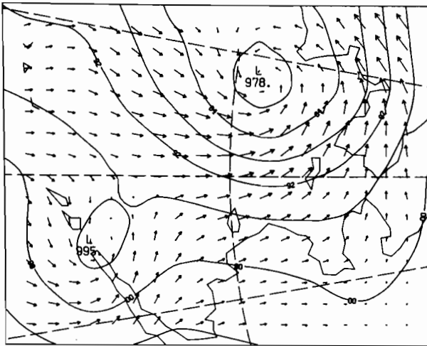
00Z 3 MAR 1981
