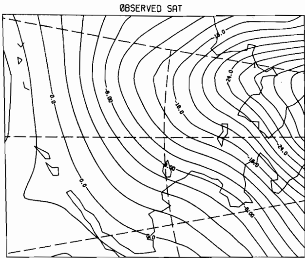
00Z 6 MAR 1981
