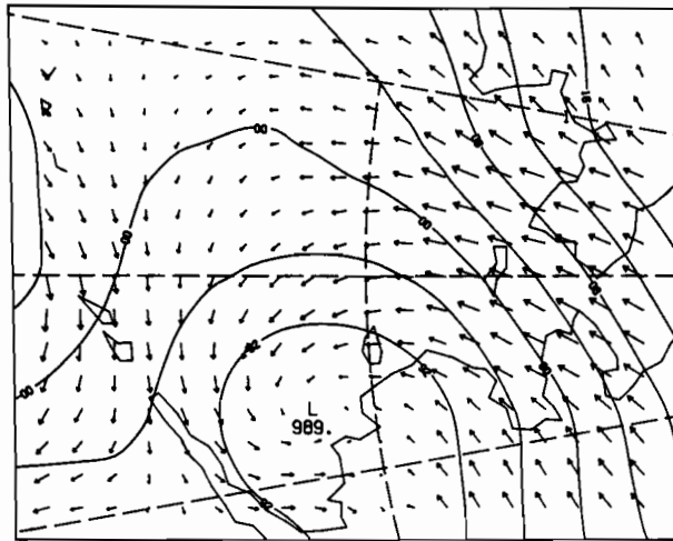
00Z 6 MAR 1981
