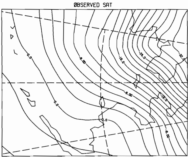
00Z 7 MAR 1981
