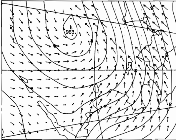
00Z 1 MAR 1981
