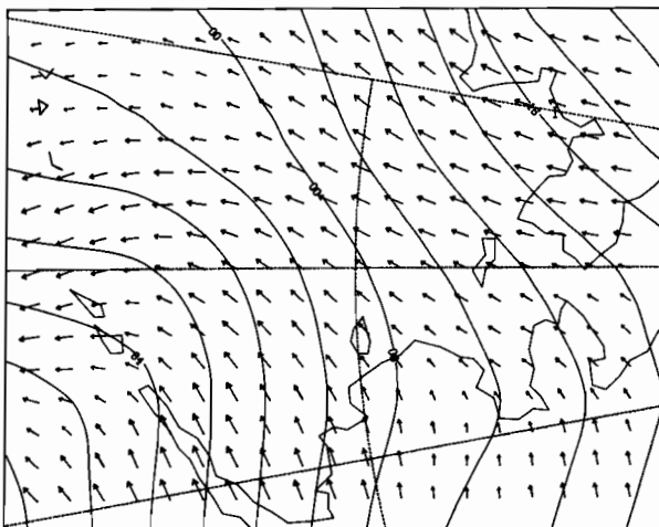
00Z 8 MAR 1981
