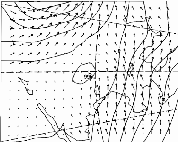
00Z 17 MAR 1981
