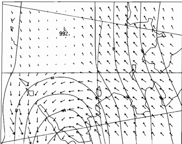
00Z 5 MAR 1981
