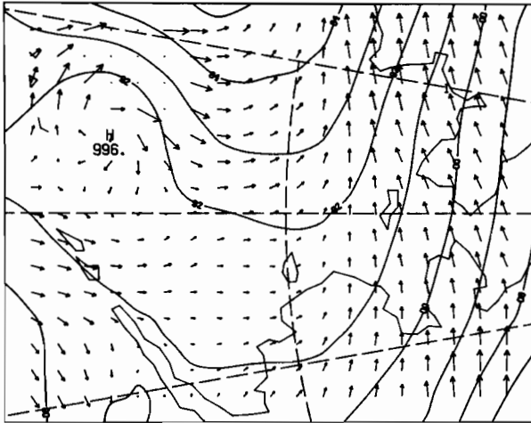
00Z 19 MAR 1981
