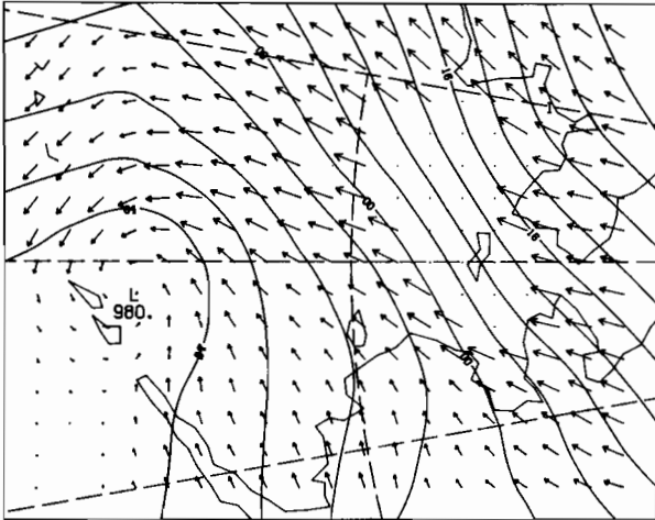
00Z 10 MAR 1981
