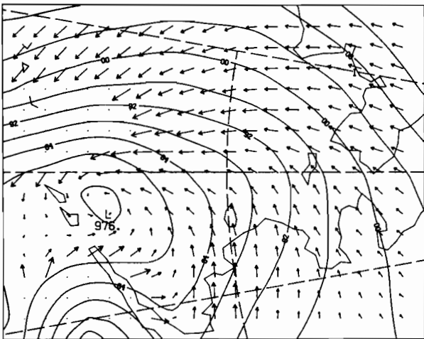
00Z 16 MAR 1981
