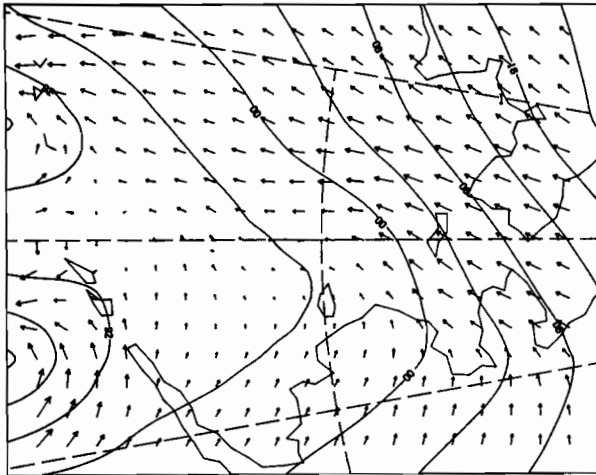
00Z 7 MAR 1981
