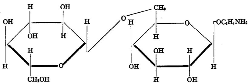
p -Aminophenol \beta -gentiobioside
