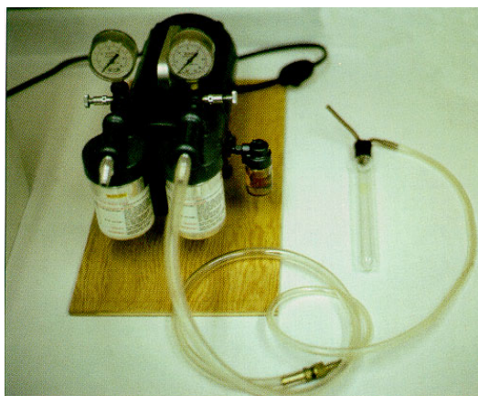
FIGURA 3-19: Ensamble del Aspirador, Mostrando la Bomba al Vacío y Tubos de Latex
