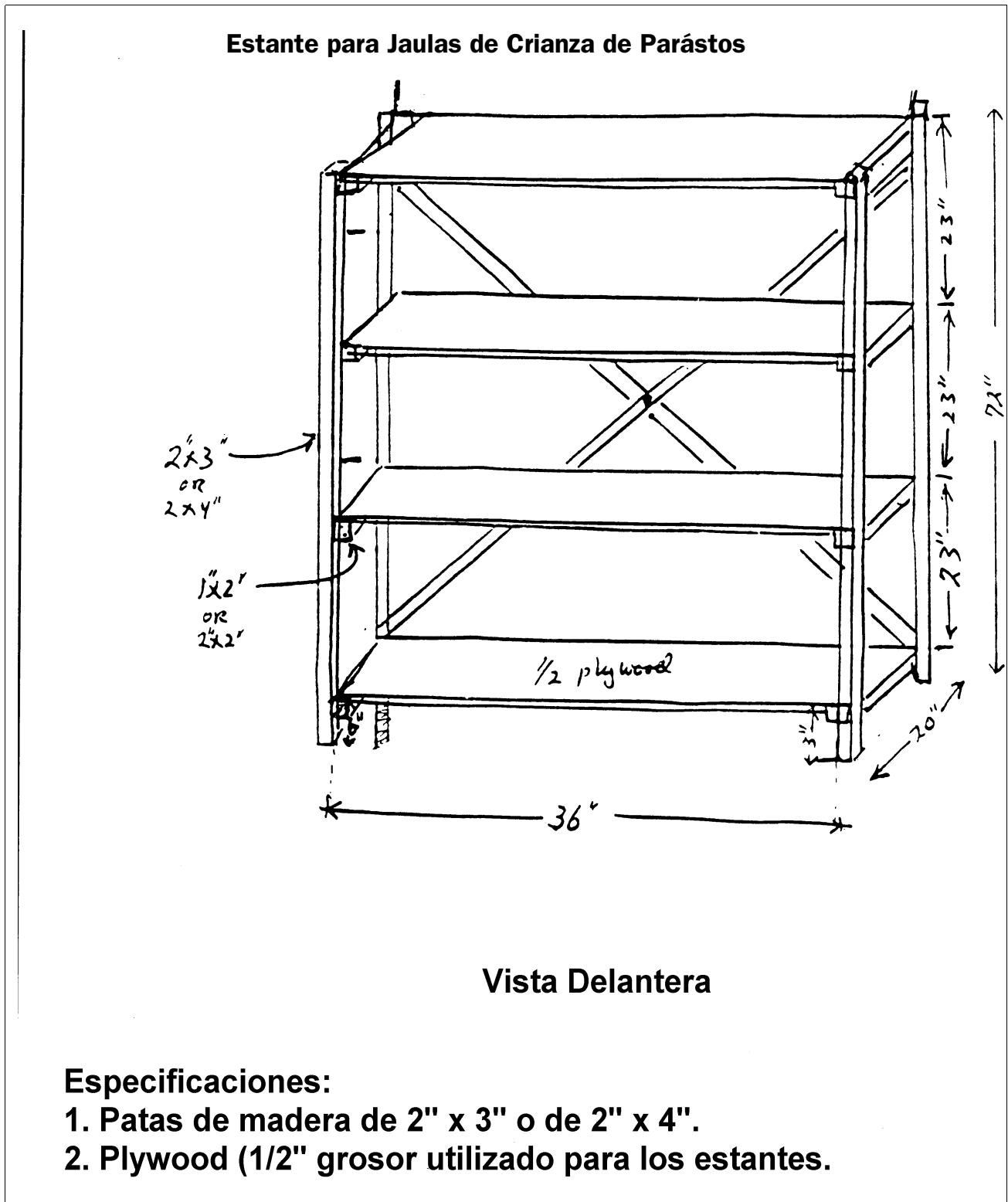
FIGURA I-2: Estante para Jaulas de Crianza de Parásitos
