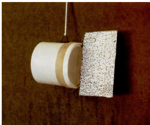
FIGURA 2-3: Trampa de Pheromona Sexual, Mostrando el Sostén de la Trampa y la Tarjeta Blanca, Pegajosa
