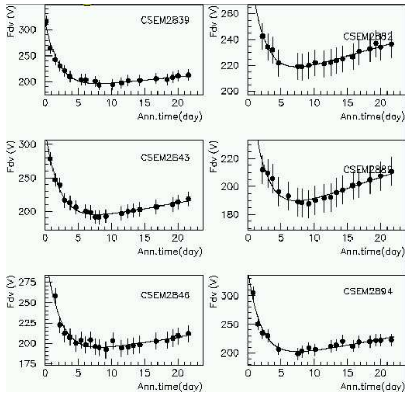
Figure 3: Tension de dépletion en fonction du temps d' annealing à 25°C. Les deux différentes périodes (bénéfique et inverse) sont bien visibles.
