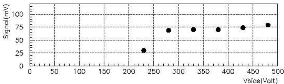
Figure 1: Signal collecté en fonction de la tension d'alimentation avec un prototype de détecteur à micro-piste en silicium irradié.
