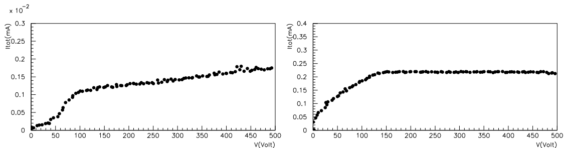
Figure 2: Caractéristique tension-courant pour le même détecteur avant et après irradiation. Les mesures ont été faites aux température de 20^{\circ}\text{C} et de -18^{\circ}\text{C} , respectivement. On observe une différence de courant de deux ordres de grandeur.
