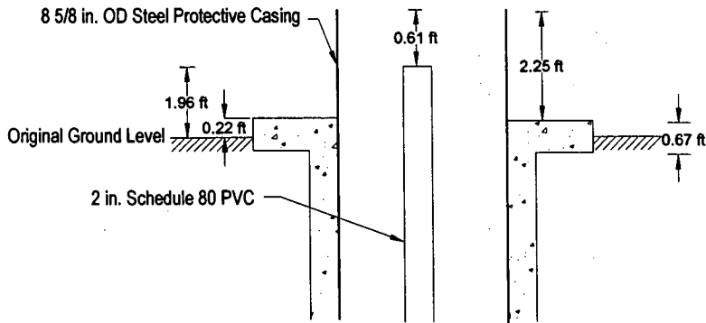
ELEVATION
