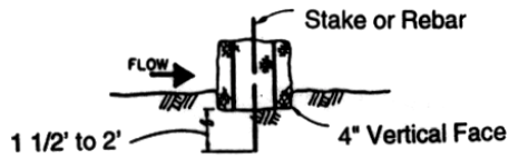
EMBEDDING DETAIL N.T.S.
