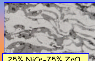
25% NiCr-75% ZrO 2
